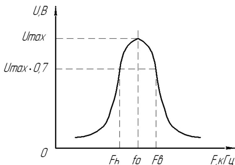
Рис. 1. Резонансний пік
