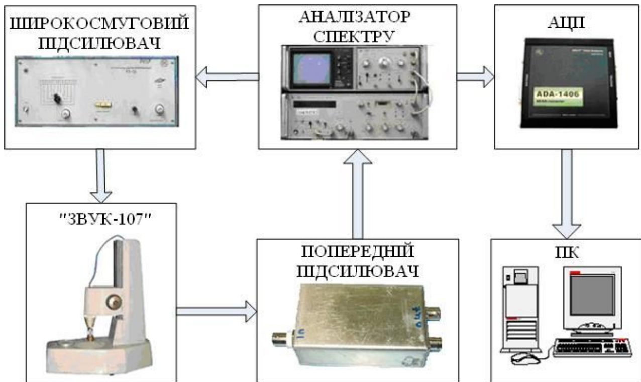
Рис.2. Автоматизована система контролю демпфуючих властивостей
