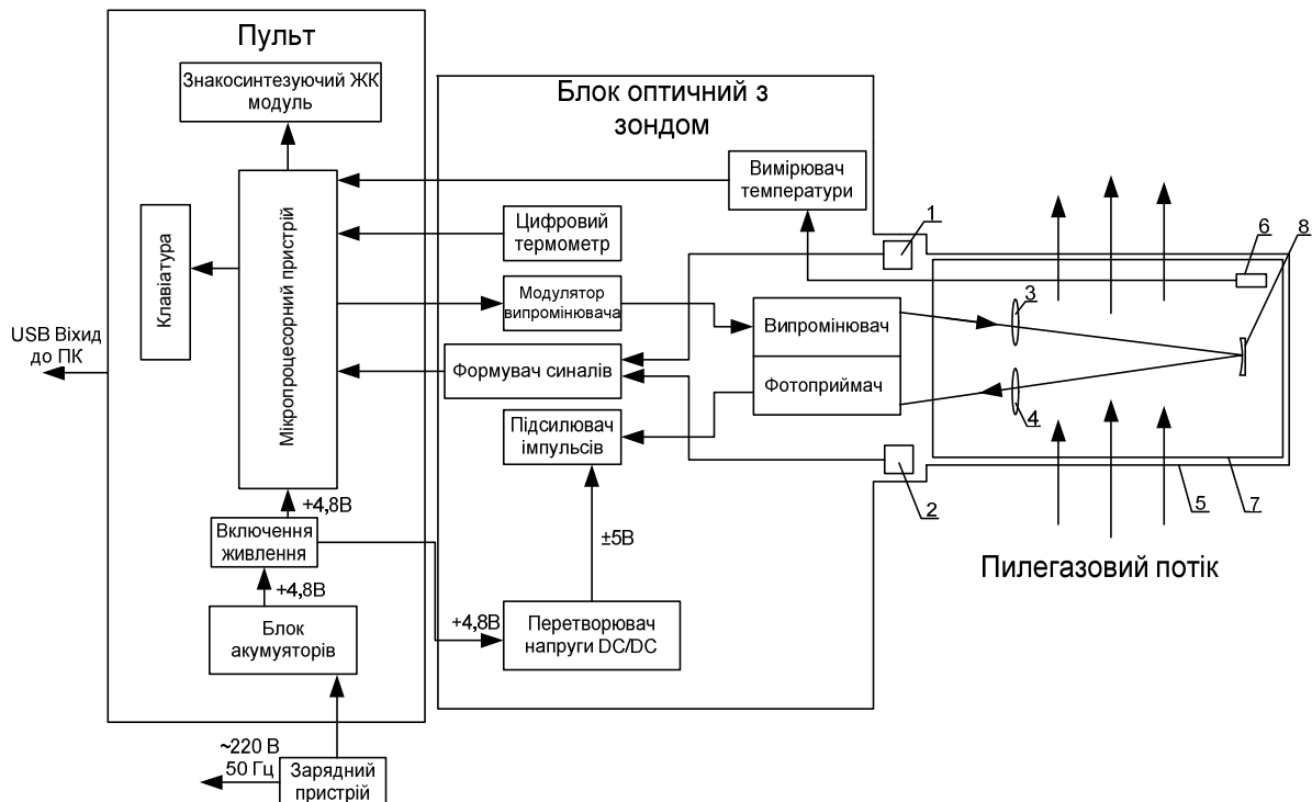
Рис. 2. Схема функціональна вимірювача ВОГ-2, де: 1, 2 – датчики положення труби-заслонки; 3 – лінза-коліматор; 4 – лінза-об'єктив; 5 – зонд; 6 – датчик температури; 7 – заслонка обертова; 8 – відбивач
